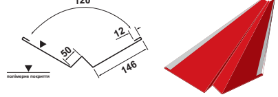
Кошикова ринва декоративна, P=312
