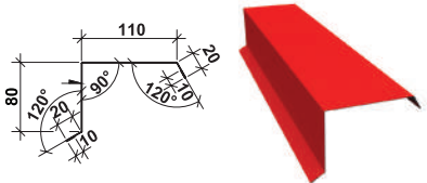
Вітрівниця верхня, P=250
