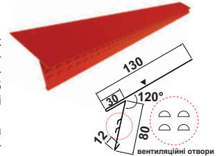
Вентиляційна карнизна планка з додатковою перфорацією, P=250
