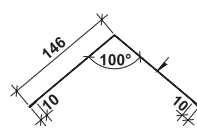
Коньок трикутний прямий, P=312
