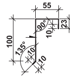
Ринва вітрова, P=125
