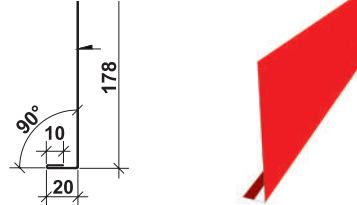
Звіс нижній, P=208
