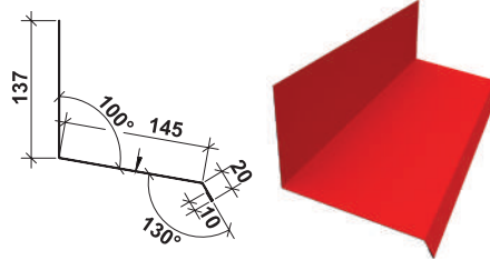
З'єднувач нижній, P=312
