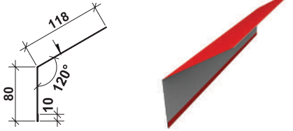
З'єднувач верхній, P=104
