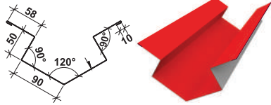
Кошикова ринва глибока, P=416
