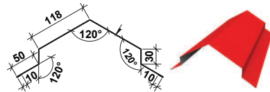
Коньок трапецієвидний, P=416
