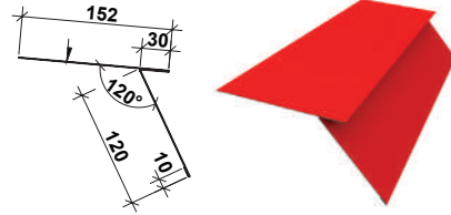
Вітрівниця верхня RetroLine, P=208
