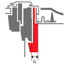
Примітка: Між віконною рамою і кроквами для каркаса утеплювача потрібно 4 см відстані з обох сторін
