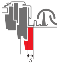
Примітка: Між віконною рамою і кроквами для каркаса утеплювача потрібно 3 см відстані з обох сторін
