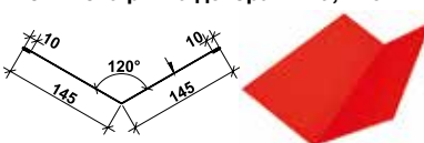
Кошикова ринва декоративна, P=312
