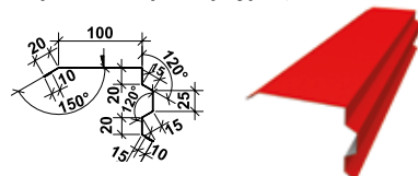
Вітрівниця верхня фігурна, P=250
