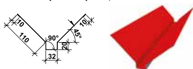
Кошикова ринва пряма, P=312
