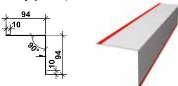
Кутник внутрішній, P=208
