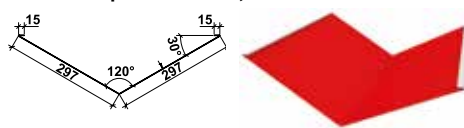
Кошикова ринва велика, P=624
