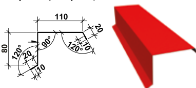
Вітрівниця верхня, P=250
