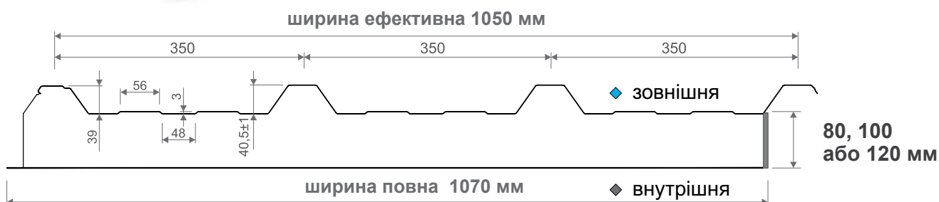
поперечний переріз
