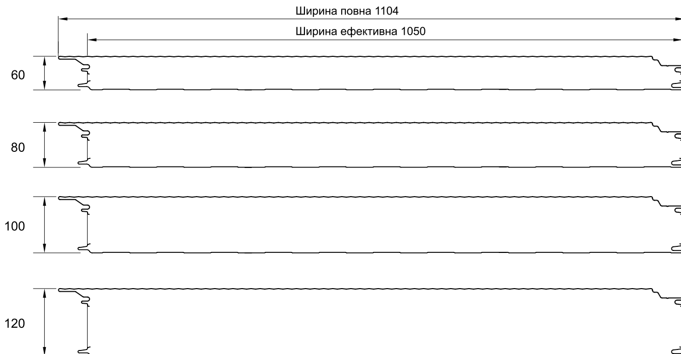
Рис. 3 Товщина панелей PWS-PIR-PL
