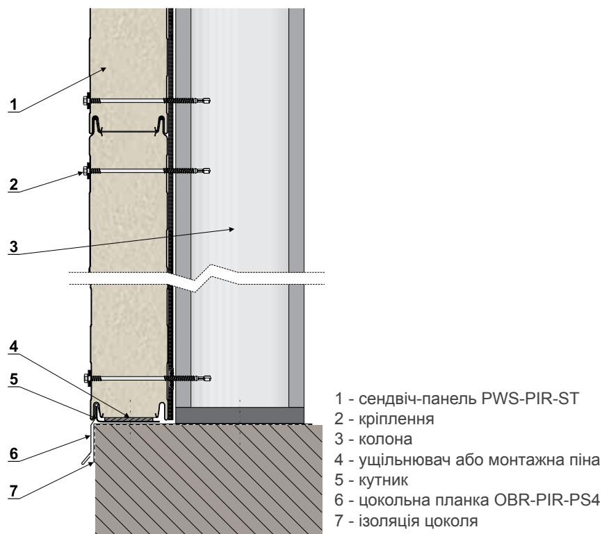
Цокольний вузол монтажу стінової сендвіч-панелі PWS-PIR ST Горизонтальний монтаж (Варіант 1)
