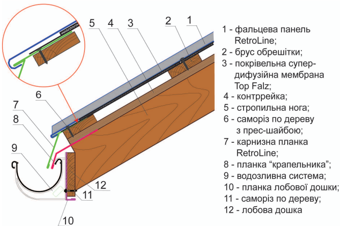
Рис.3. Схема монтажу панелей RetroLine з використанням супердифмембрани TOP FALZ
