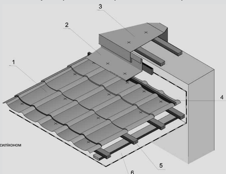
Рис. 16. Вузол примикання покрівлі до стіни по торцю
