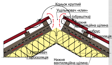
Коньковий вузол із застосуванням плівки з низькою паропроnikною здатністю (гідробар'єр) (вершина не обшита плівкою)
