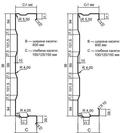
Стінова касета
