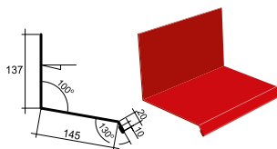
З'єднувач нижній, P=312
