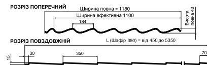
ШАФІР 350
