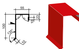
Ринва вітрова, P=125
