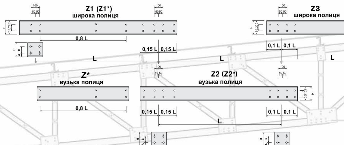
Монтажна схема прогонів для прольотів L > 6000
