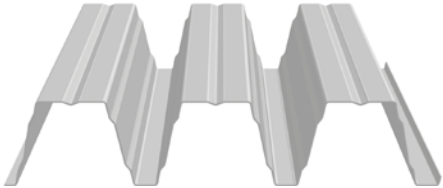
T160 \neq 0,75–1,5 мм — макс. довжина 13,6 м
