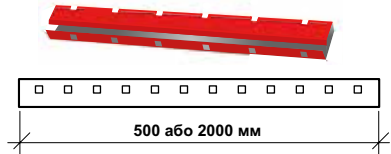
Підконькова планка RetroLine (IRYD та KARPATIA) P=137,5
