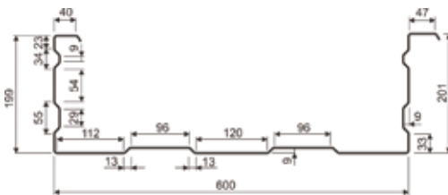
Стінова касета
