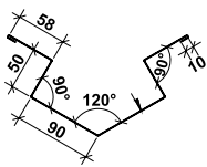
Кошикова ринва глибока, P=416
