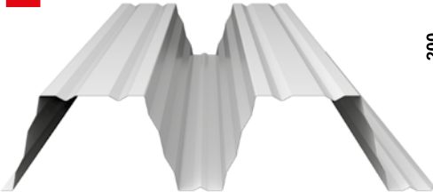
T200 \neq 0,75–1,5 мм — макс. довжина 13,6 м
