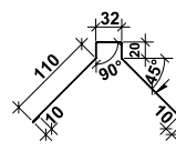
Коньок прямиий, P=312
