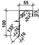
Ринва вітрова, P=125
