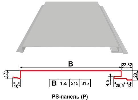
PS-панель (P)
