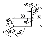
З'єднувач малий, P=208
