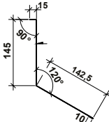
З'єднувач великий, P=312
