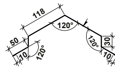
Коньок трапецієвидний, P=416
