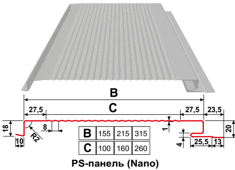
PS-панель (Nano)
