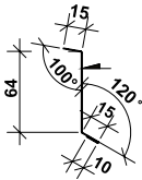
З'єднувач верхній, P=104
