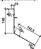
Кошикова ринва велика, P=624
