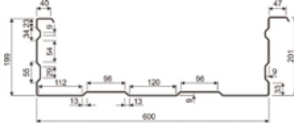
Стінова касета глибиною 200 мм
