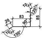
З'єднувач малий, P=208
