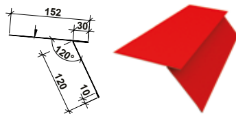
Вітрівниця верхня RetroLine, P=208
