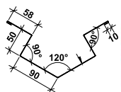
Кошикова ринва глибока, P=416
