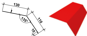
Вітрівниця верхня ARAD, P=156
