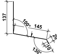
З'єднувач нижній, P=312
