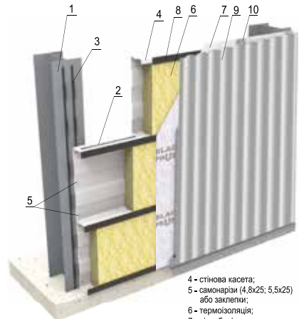
Стінова касета стартова
