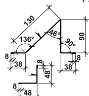
Кутник внутрішній СБ, P=112
