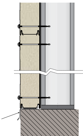
Цокольний вузол Горизонтальне розташування Варіант 1
