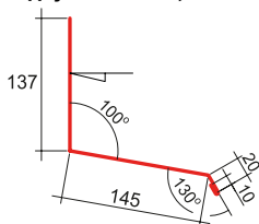
З'єднувач нижній, P=312
