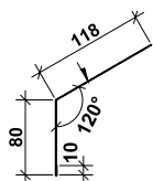
Звіс верхній, P=208
