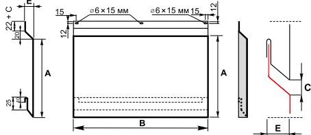
Касетон К-2
