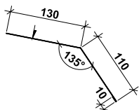
Вітрівниця верхня ARAD, P=156
