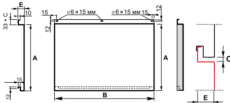
Касетон К-2
