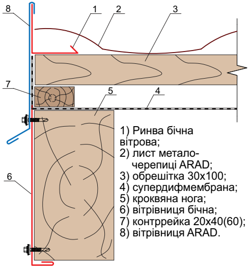
Рис. 2.1. Вітровий вузол
