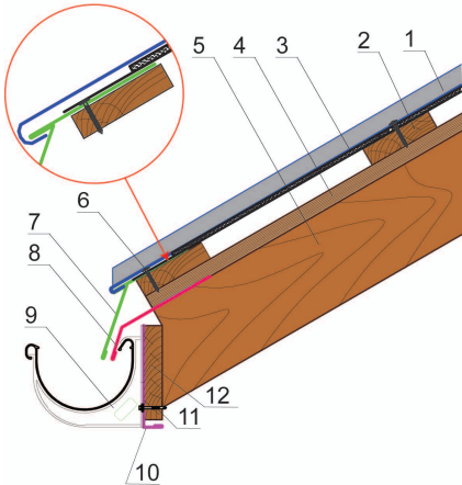
Рис.3. Схема монтажу панелей RetroLine з використанням супердифмембрани TOP FALZ
